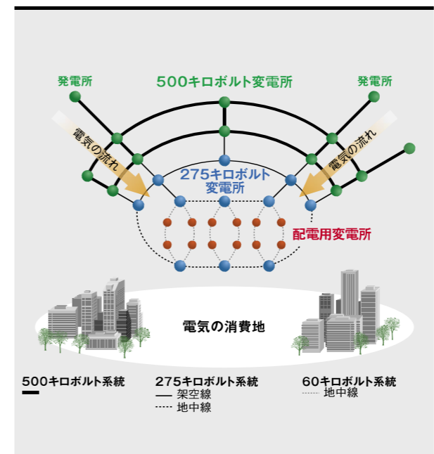
図 8.17.2 東京電力の電力系統
